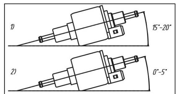
Rys. 22. Kąt montażu pompy paliwa TH-9; TH-10; TH-11 (1) i pompy paliwa Thomas Magnete (2).
